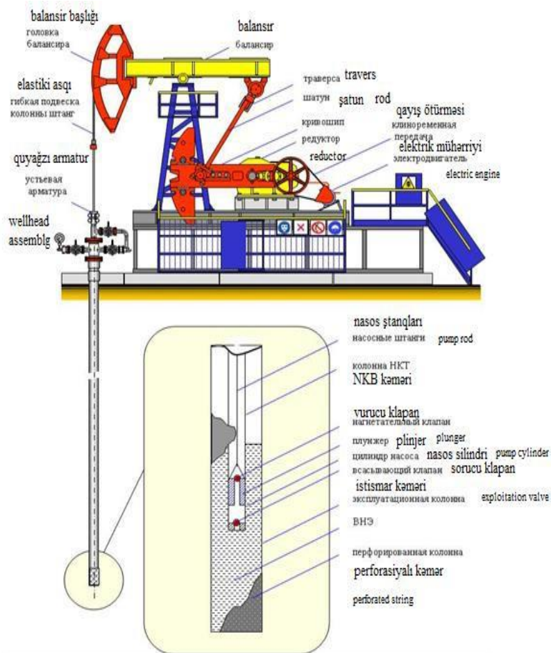
Neftçixarma üçün mancanaq dəzgahının sxemi Схема станок качалки для нефтедобычи Diagram of beam pumping for oil production
